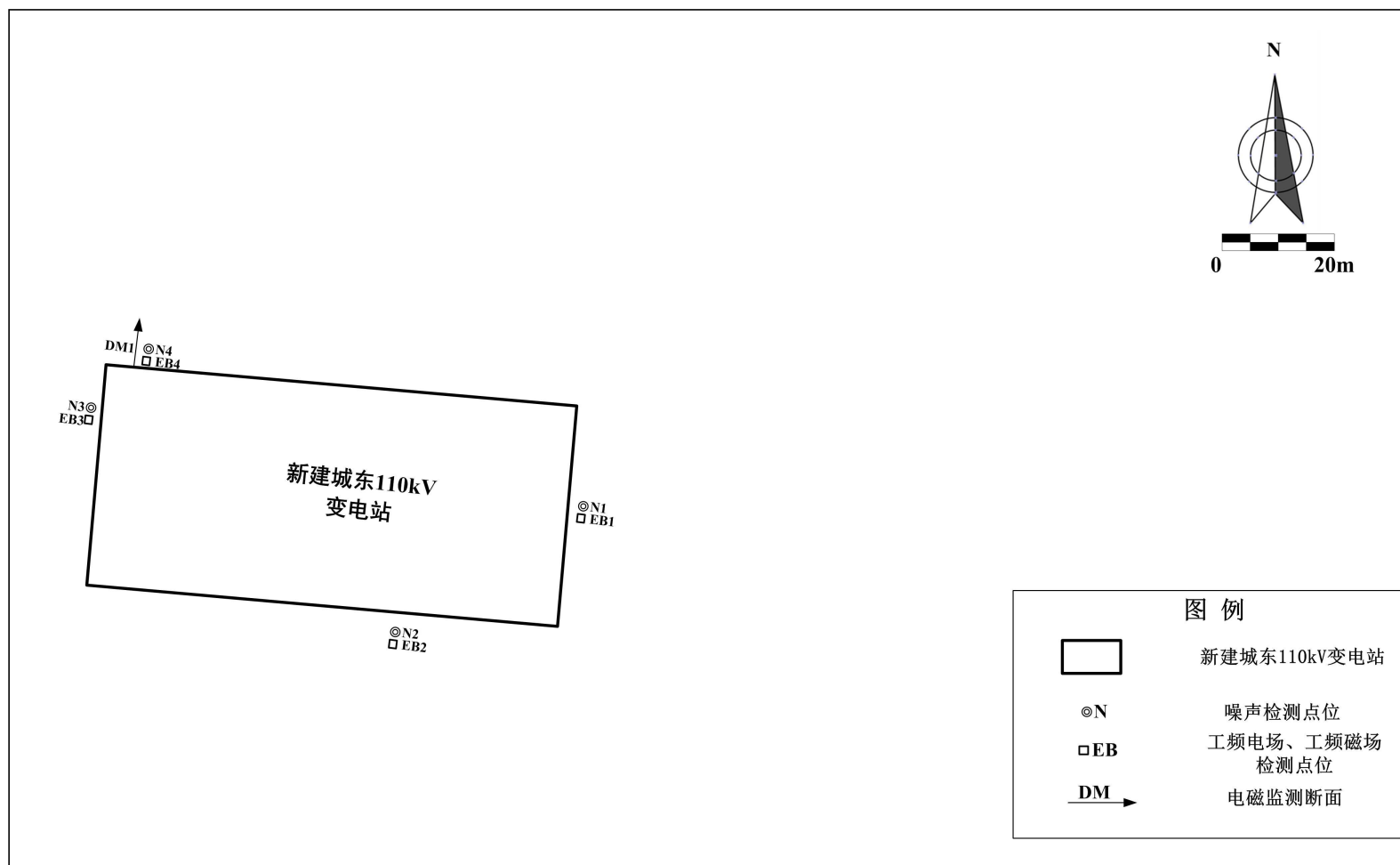
图 7-1 城东 110kV 变电站电磁环境及声环境监测点位示意图
