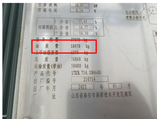
#2 主变油量
