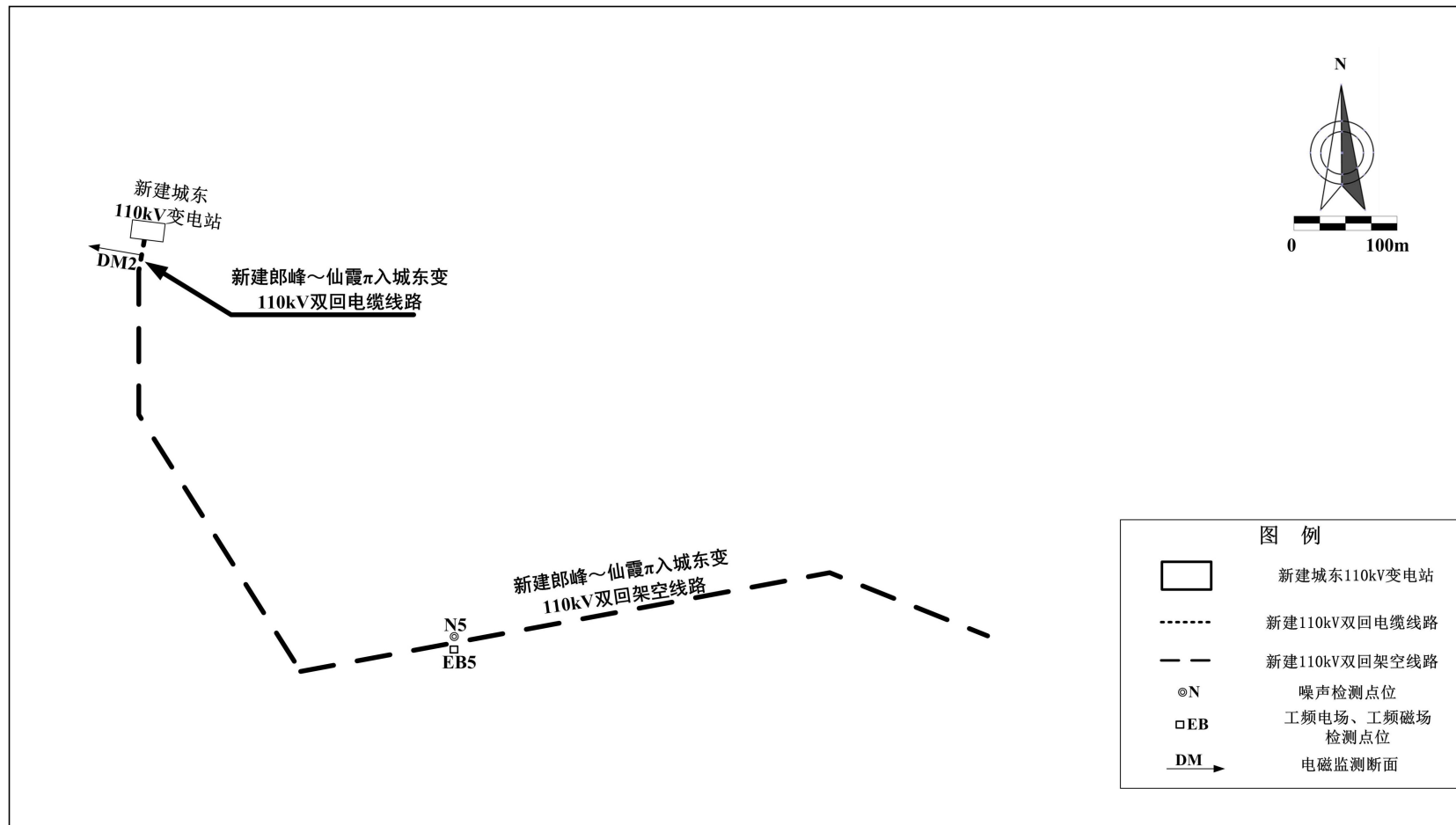
图 7-2 本项目输电线路电磁环境及声环境监测点位示意图
