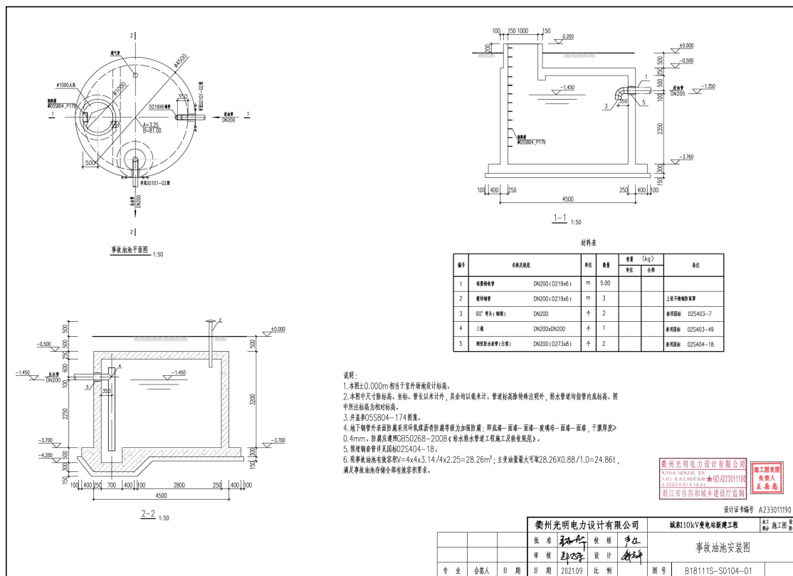
城东110kV变电站事故油池结构图见图8-2。
