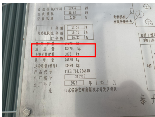
#1 主变油量
