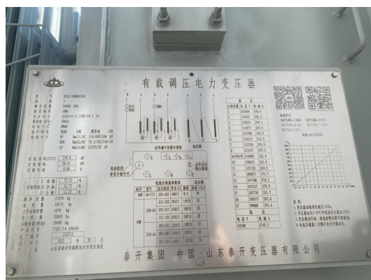
#1 主变铭牌
