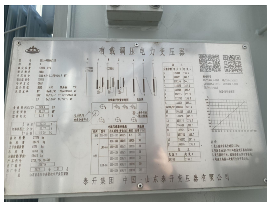
#2 主变铭牌
